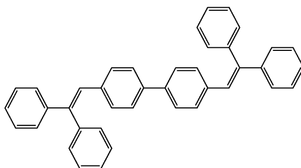
DPABi
